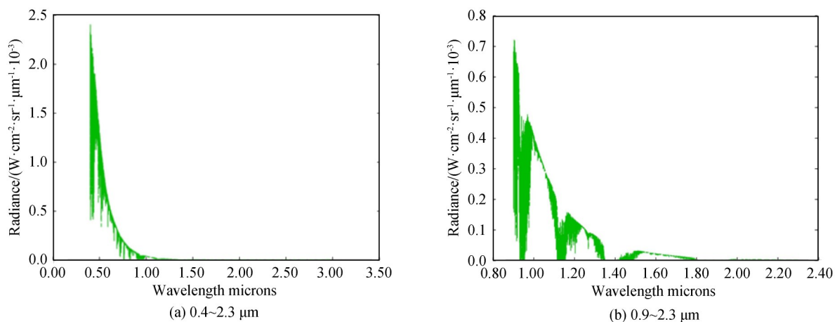
图4 天空背景光谱辐射亮度
