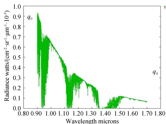
图6 天空背景辐射
