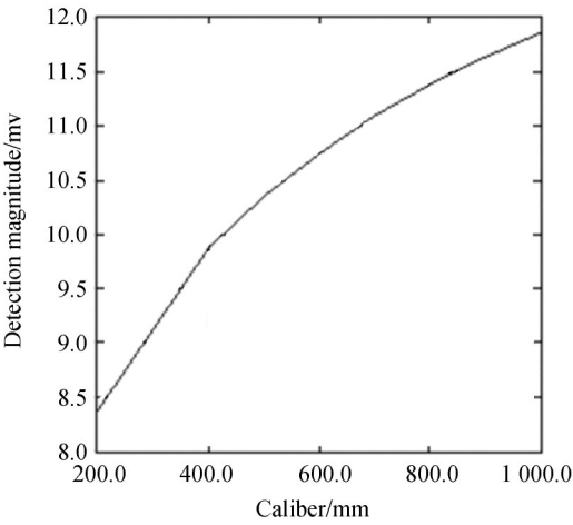
图 8 探测星等与口径的关系
