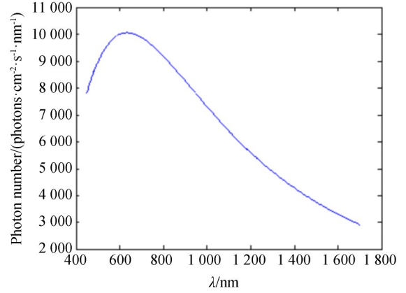
图 1 0 等星太阳光谱光子数
