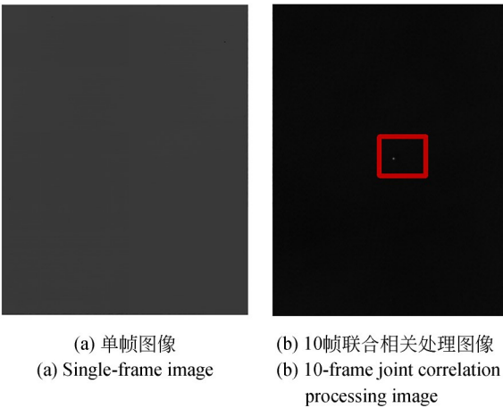
图 10 恒星编号 13017 的观测效果 Fig. 10 Observation results of star number 13017
