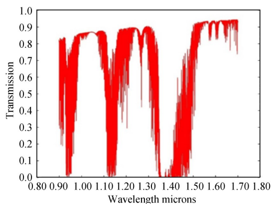
图5 大气透过率
