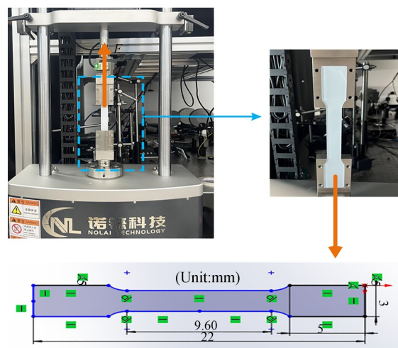
图2 被测玻璃及夹持拉伸实物
