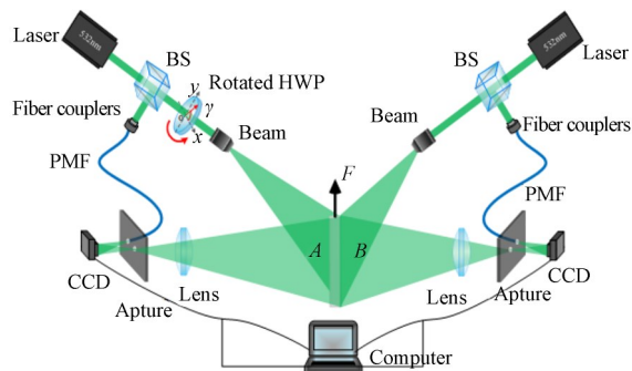
图3 数字散斑干涉双光路测量系统
