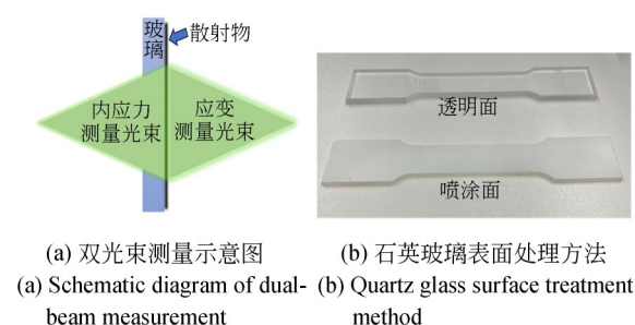
图1 对向双光路测量原理及试件表面处理
