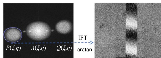
图9 空间频谱及高频项相位分布
