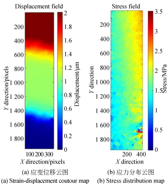
图 11 系统测量结果
