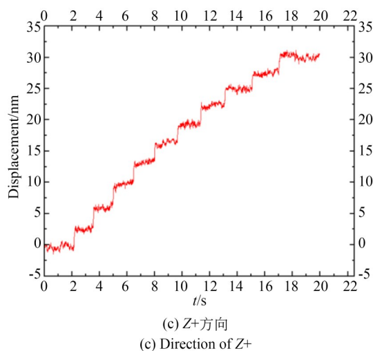
图10 各向接触时测球相对位移
