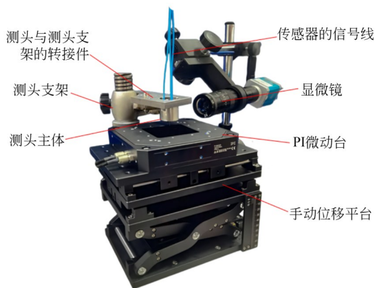
图9 测头测试平台
