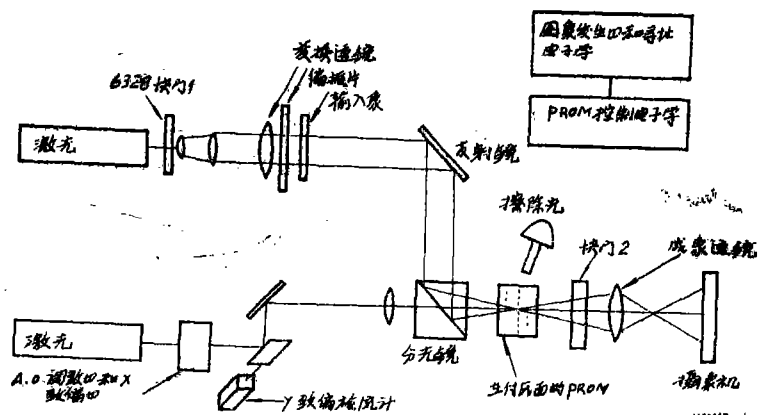
图17 利用一个 PROM 的计算机控制付氏面的滤波系统示意图
