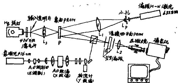
图19 利用 PROM 装置的复杂光学处理系统
