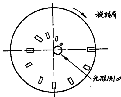
图3 在混合光学/电子学测量系统中做为角度函数的衍射强度测量的旋转屏
