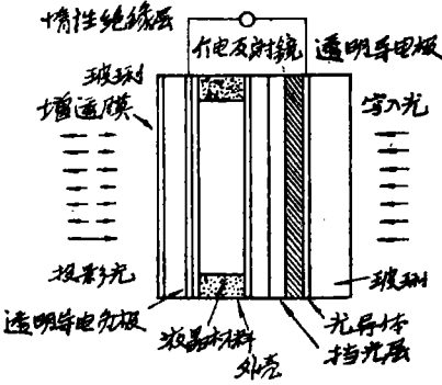
图13 交流(ac)液晶装置示意图
