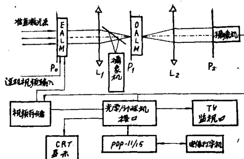
图22 混合的光学—数字处理器的框图
