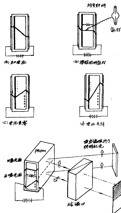
图11 PROM 装置工作示意图
