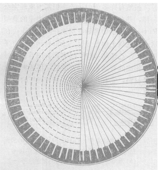
图6 直径1.25吋扇形探测器，带有32个楔形元件和32个半圆环
