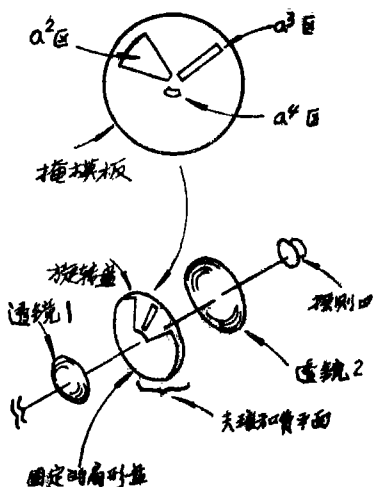
图4 粒子分布特性的衍射测量。光学系统表示出了固定和旋转的掩模板
