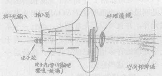
图15 电子束寻址油膜装置的示意图
