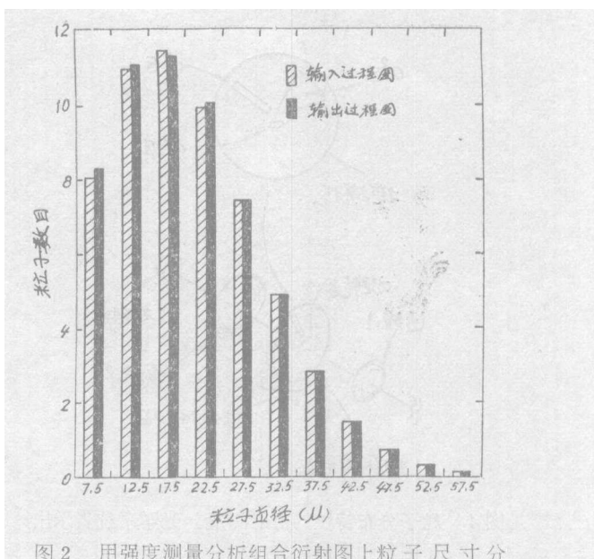
图2 用强度测量分析组合衍射图上粒子尺寸分布。这里给出的检验之例是比较输入和输出过程图(histogram)信息
