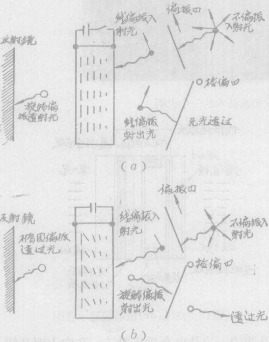
图14 液晶装置的工作 (a)断态 (b)通态
