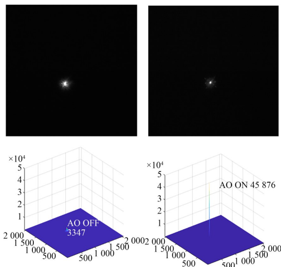
图 16 校正前(左)校正后(右)的光源成像效果对比
