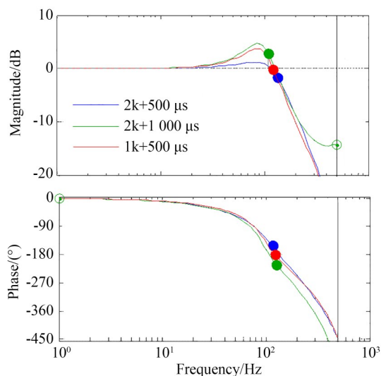
图 3 控制环路闭环频率特性曲线
