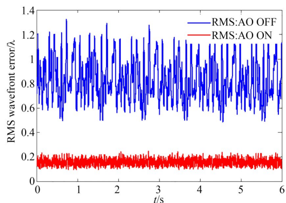
图 18 校正前后系统的波前残差曲线
