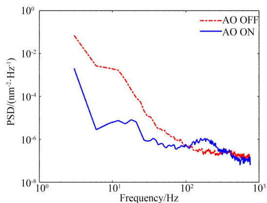
图 17 校正前后系统波前残差功率谱
