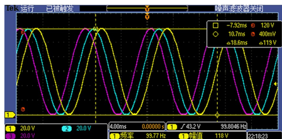
图 15 DA 转换器为模拟源的高压放大器响应曲线
