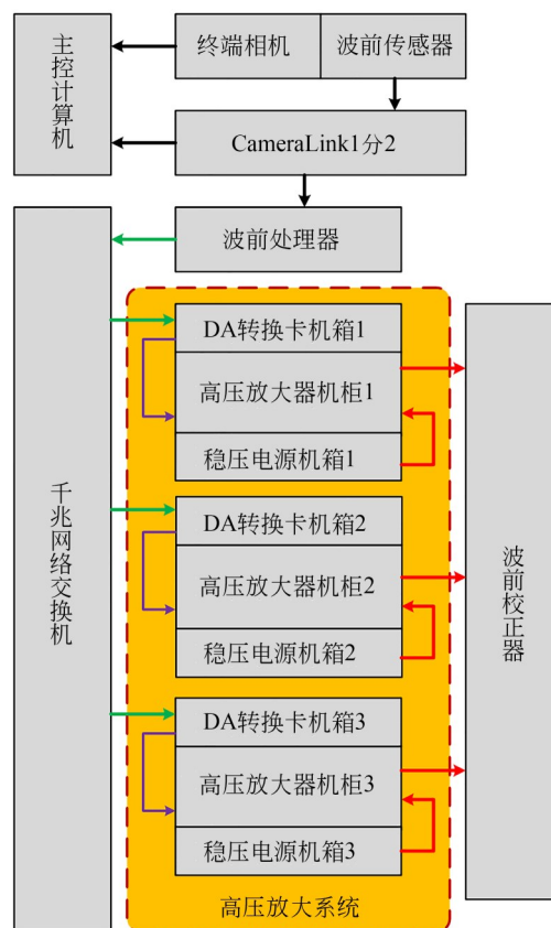
图 10 自适应光学系统电控部分集成框图
