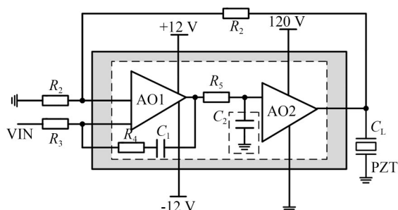
图 9 高压放大器的两级放大结构框图
