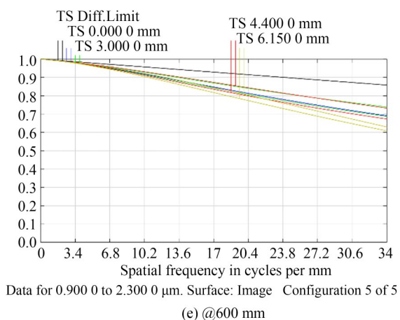
图 5 不同工作距离处光学系统的 MTF 曲线
